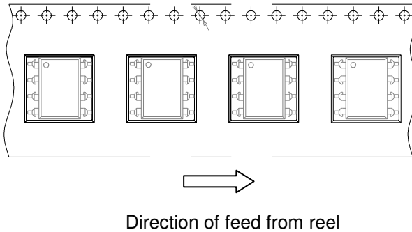
Option TA
